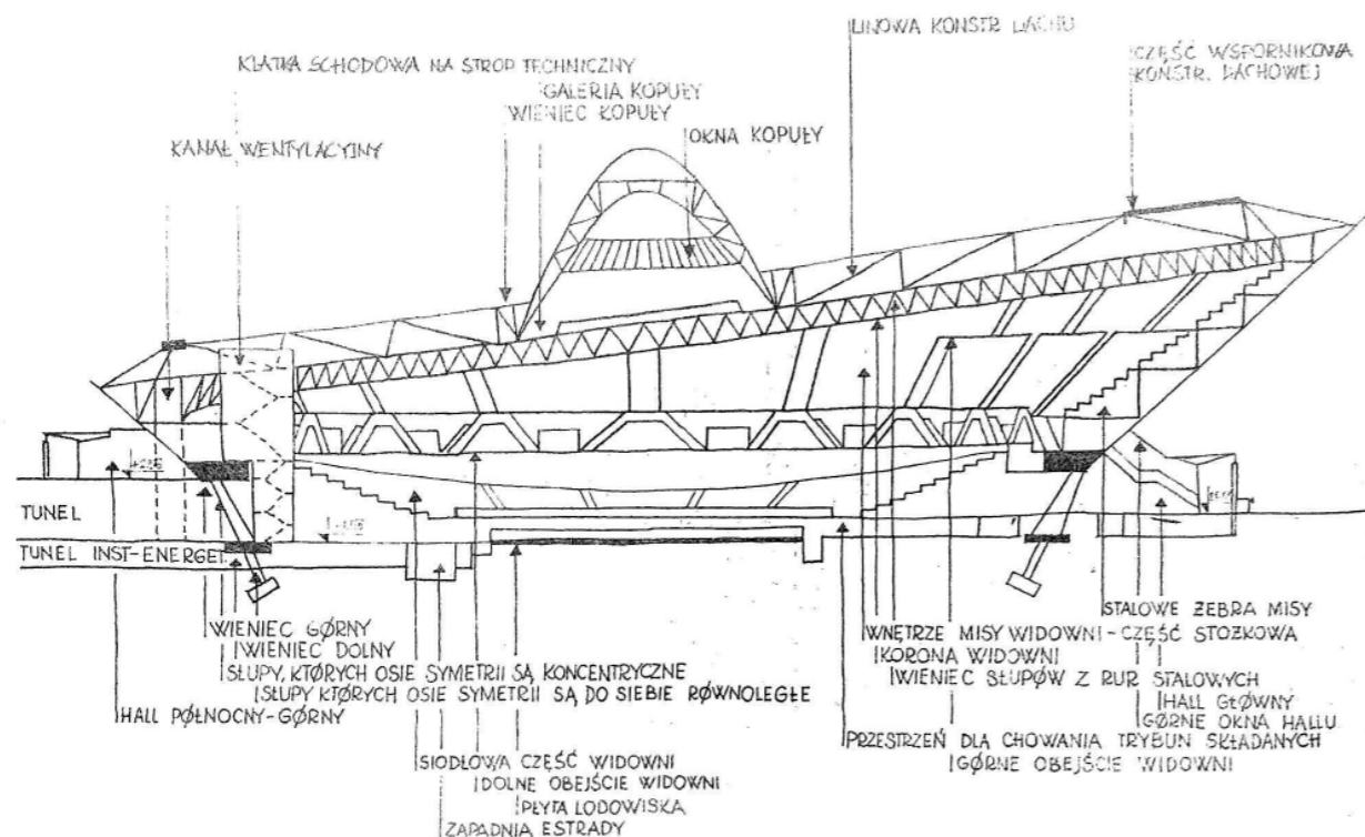
► Schemat przekroju hali głównej
